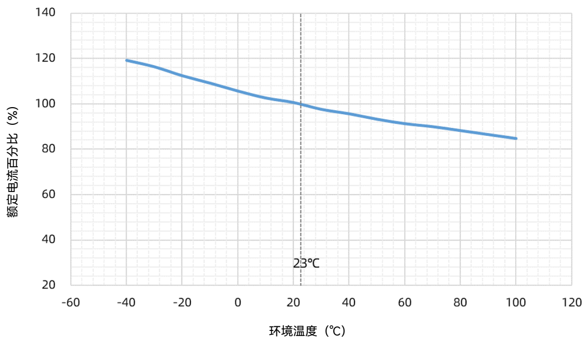
SHP 45 A 降额曲线
