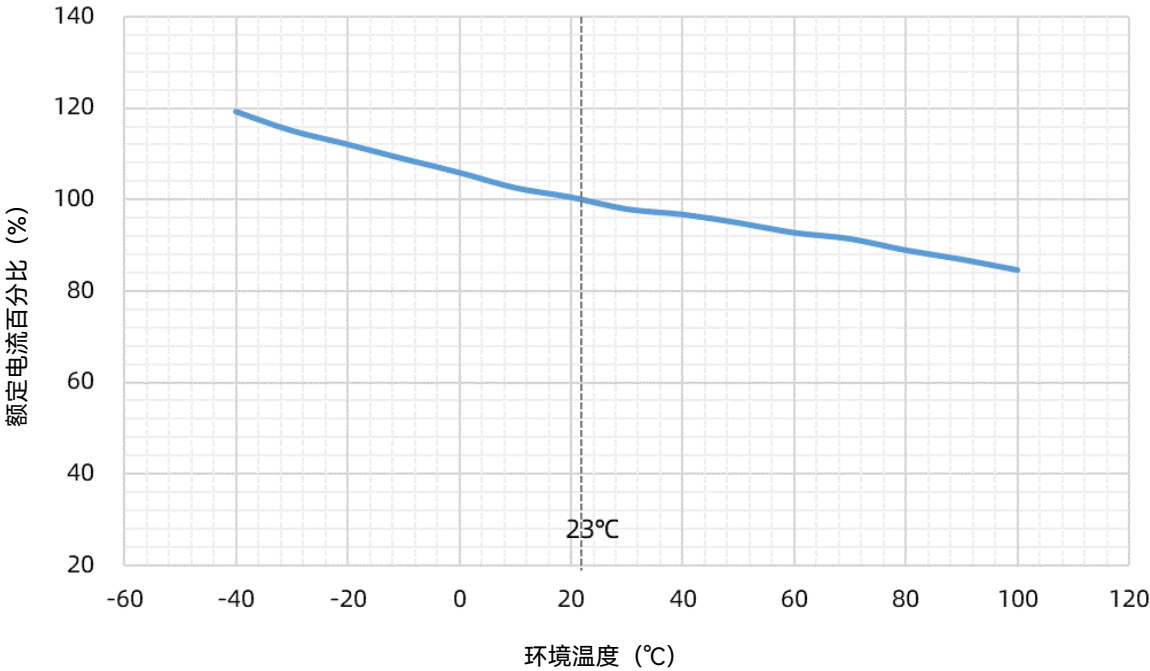
SHP 60 A 降额曲线
