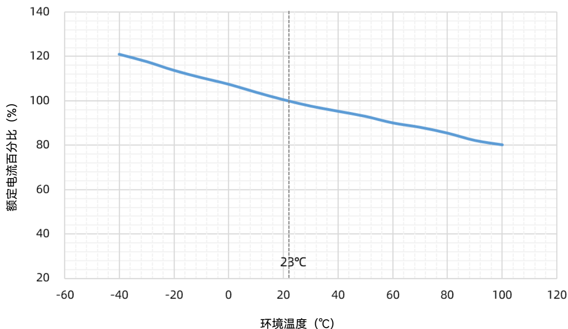
SHP 30 A 降额曲线
