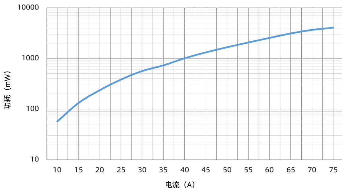
SHP 75 A 电流-功耗曲线
