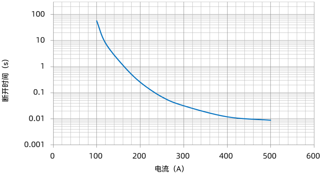
SHP 60 A 电流-时间曲线
