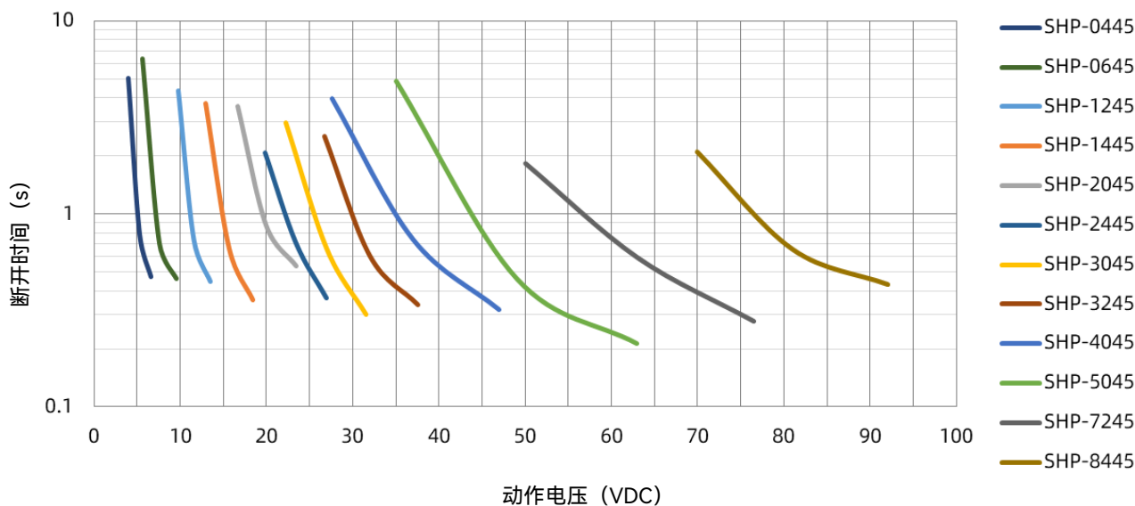
SHP 45 A 受控熔断时间曲线
