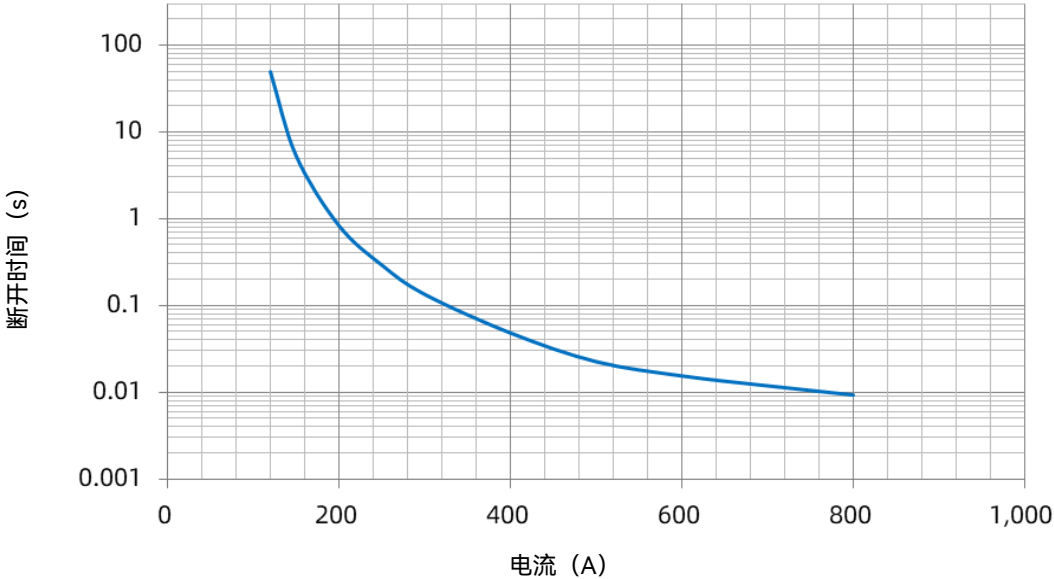
SHP 75 A 电流-时间曲线
