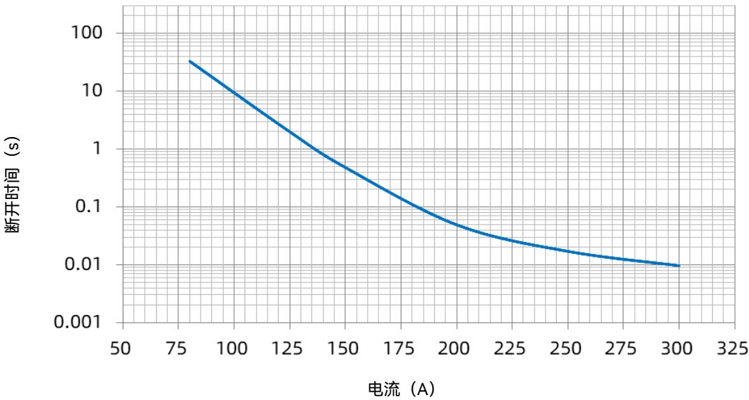
SHP 45 A 电流-时间曲线
