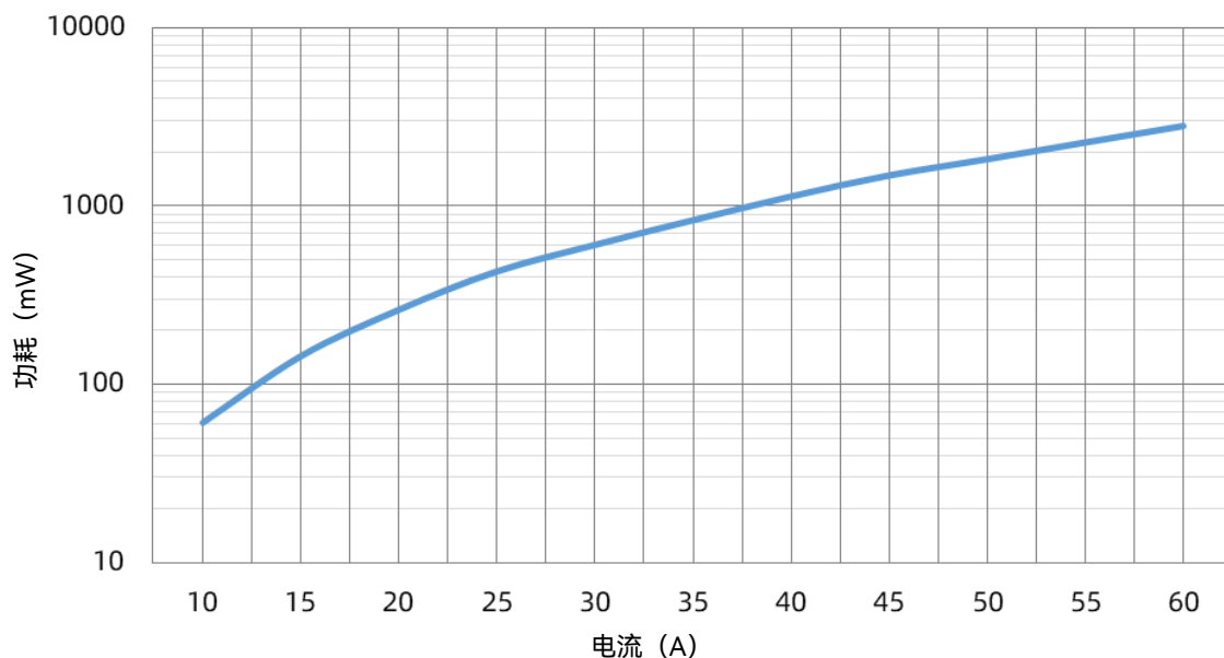
SHP 60 A 电流-功耗曲线
