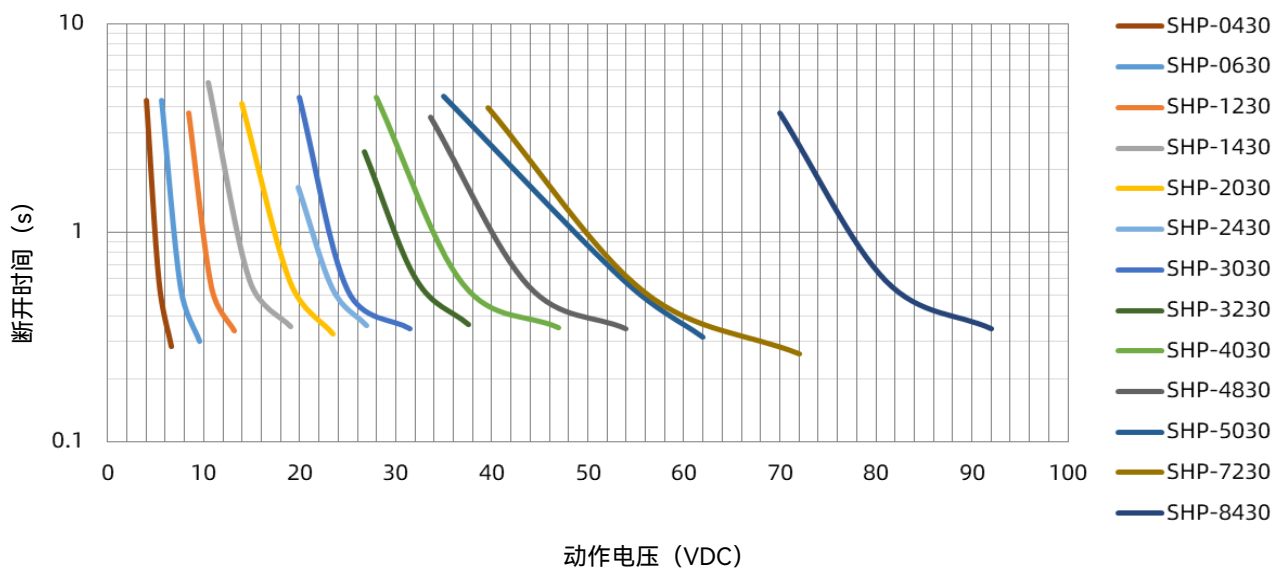
SHP 30 A 受控熔断时间曲线
