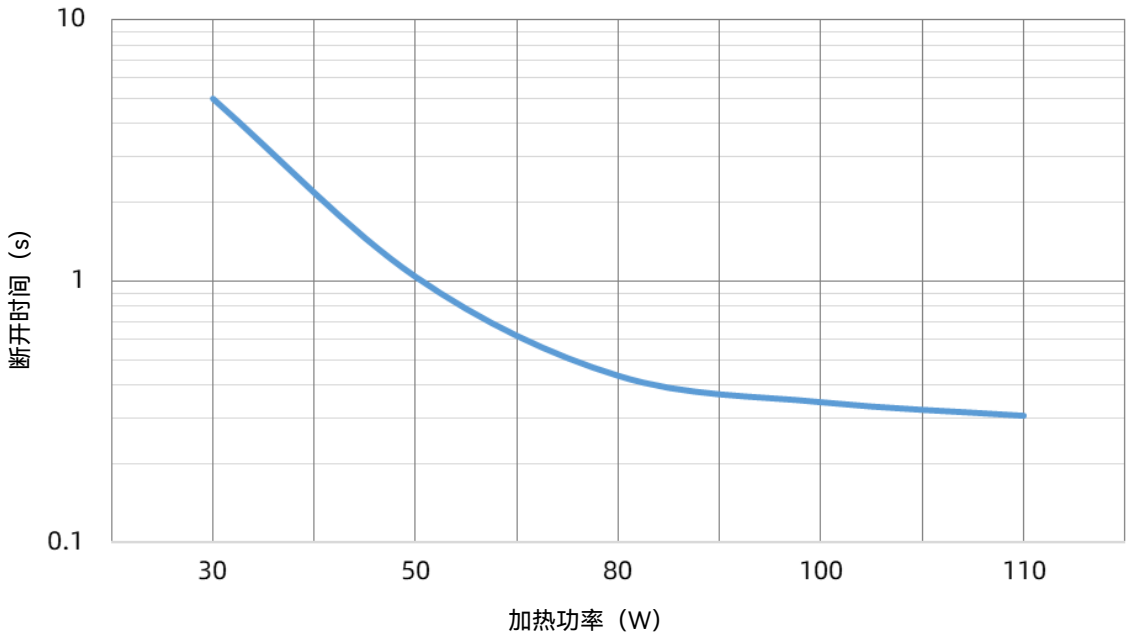
SHP 30 A 功率-时间曲线
