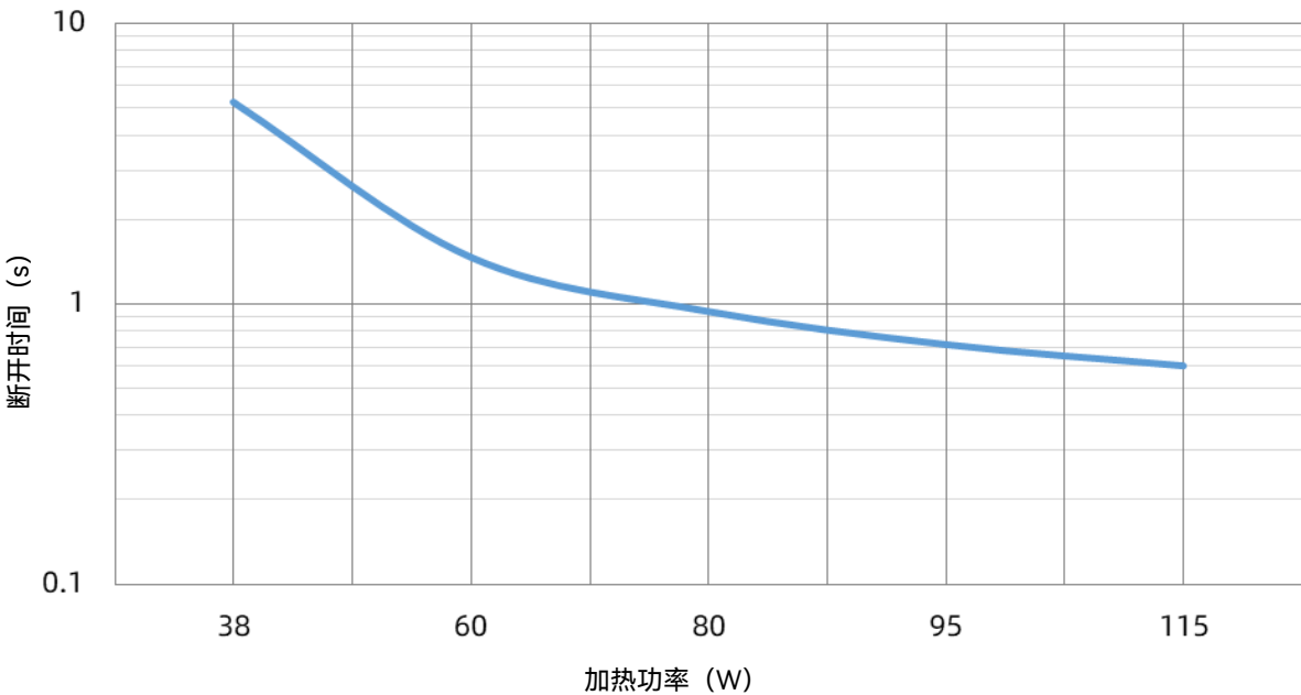
SHP 60 A 功率-时间曲线
