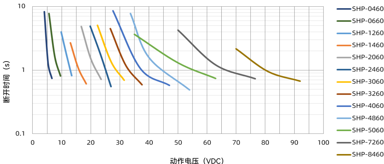
SHP 60 A 受控熔断时间曲线
