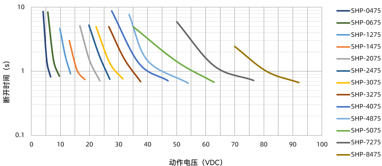
SHP 75 A 受控熔断时间曲线
