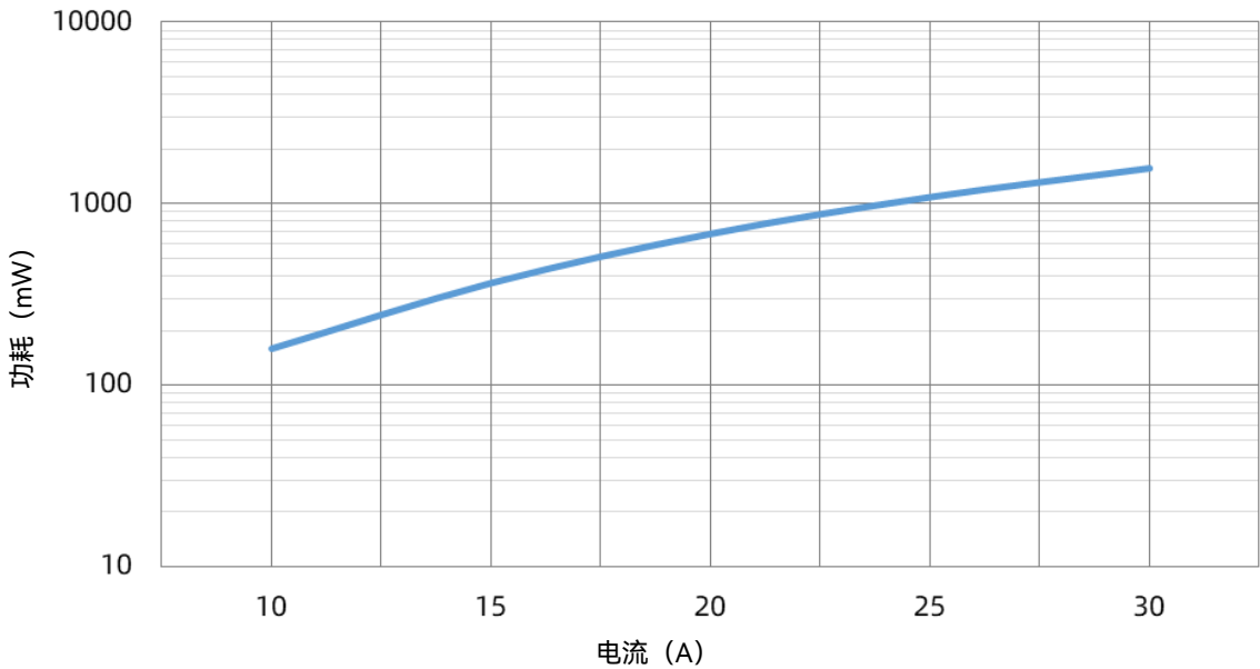
SHP 30 A 电流-功耗曲线
