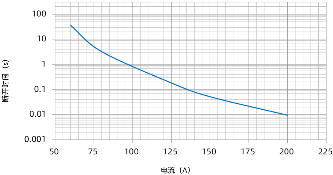
SHP 30 A 电流-时间曲线
