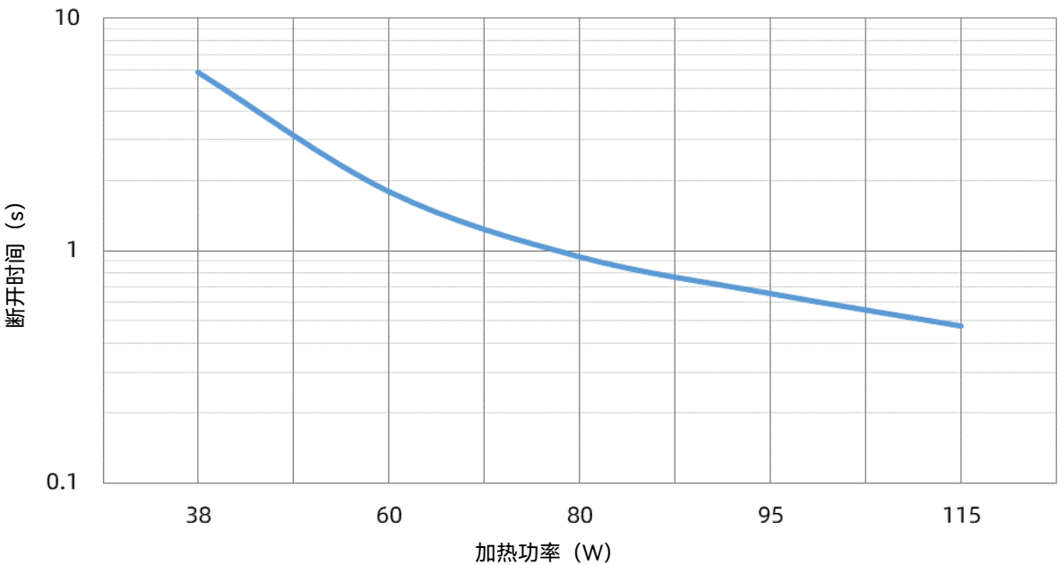
SHP 75 A 功率-时间曲线
