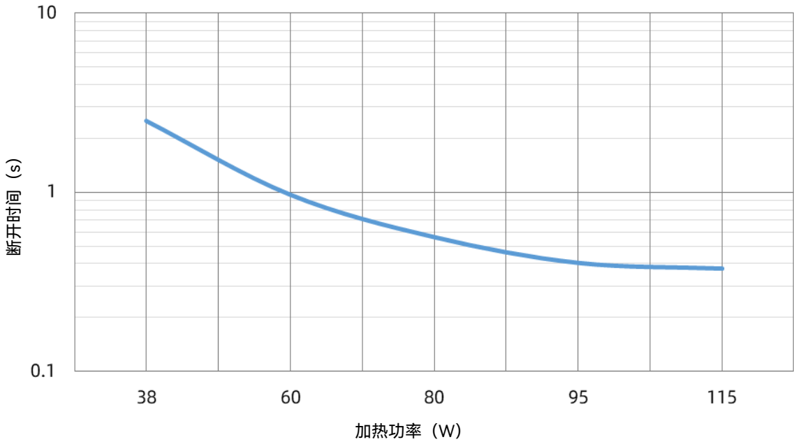
SHP 45 A 功率-时间曲线
