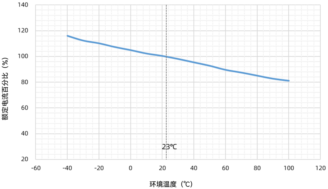
SHP 75 A 降额曲线
