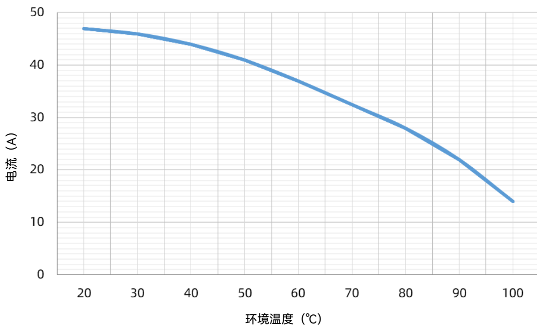
SHP 45 A 载流能力曲线
