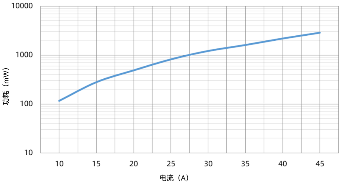
SHP 45 A 电流-功耗曲线
