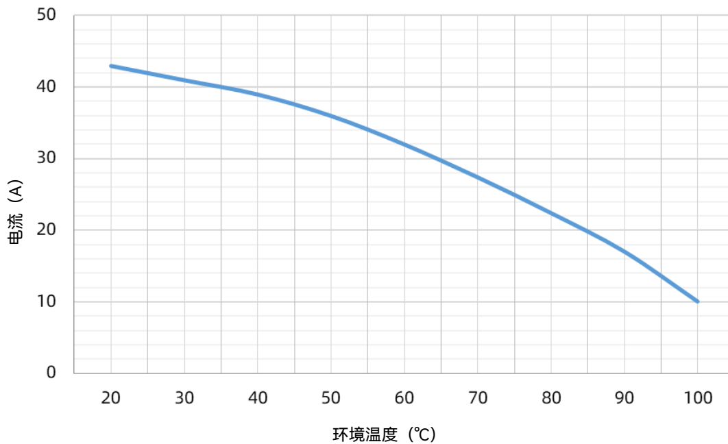
SHP 30 A 载流能力曲线
